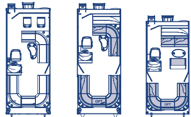
2080-P 6,7-2,59-P 2080-D 6,7-2,59-B 1880-B 6,7-2,59-B pieds mètres
